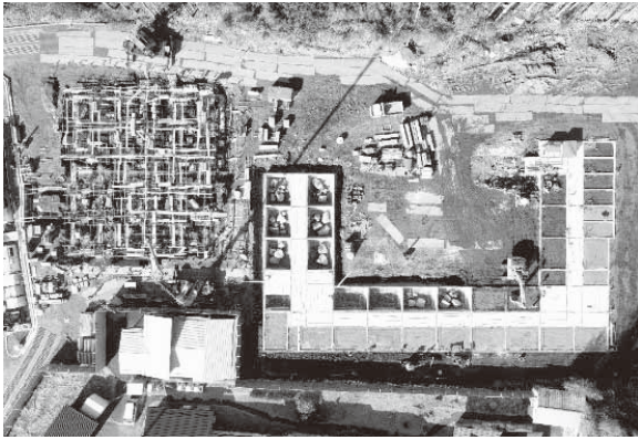
上空から見た 基礎工事施工状況
