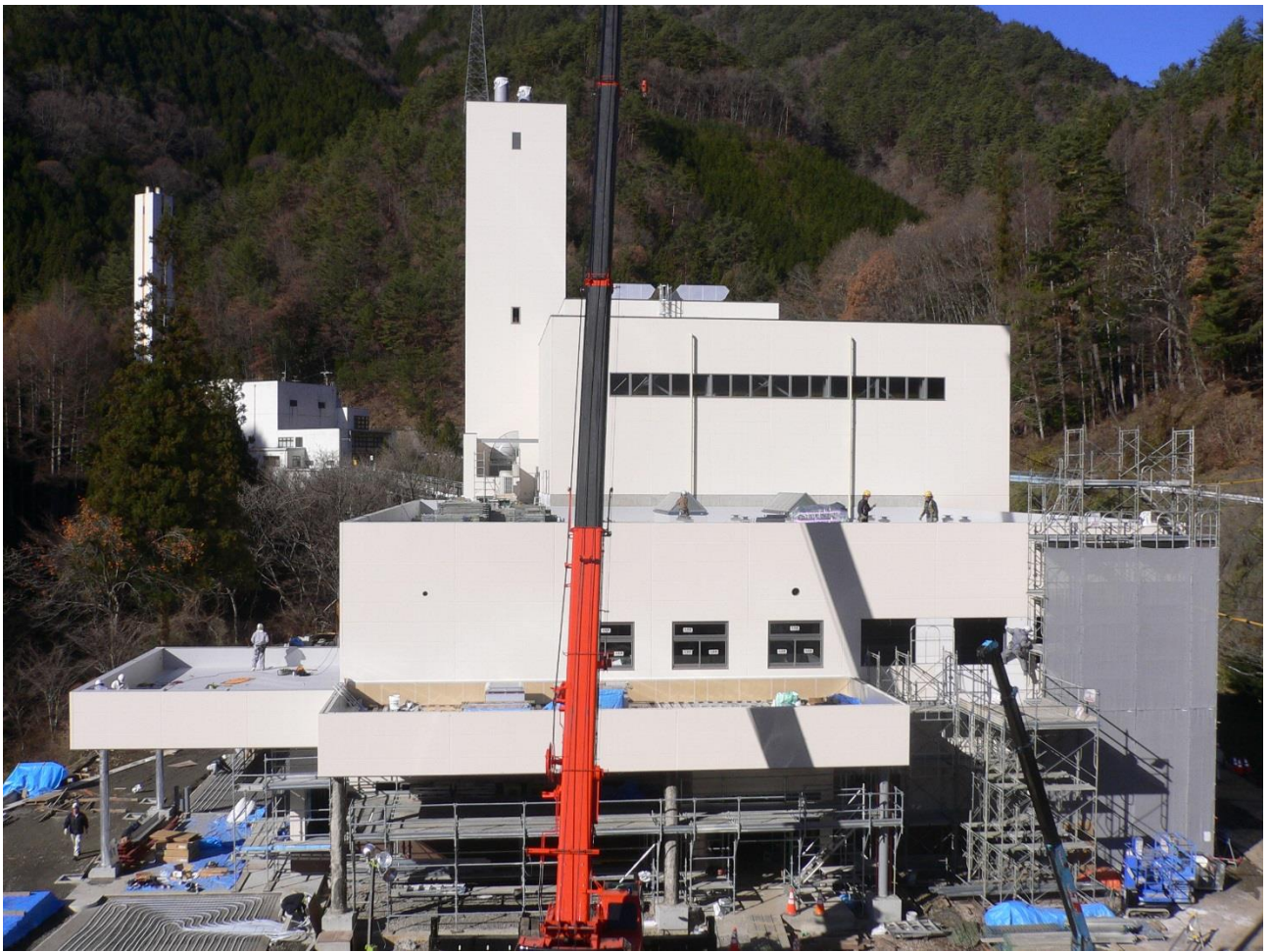
新ごみ処理施設の全景（平成 29 年 11 月 21 日 南側より撮影）
